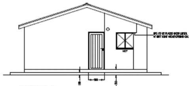
ELEVATION - 3
